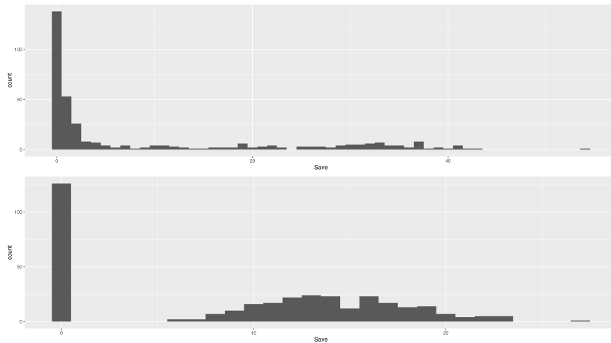
図 6.9 ゼロ過剰ポアソン分布による当てはめ。上がロウデータ, 下が事後予測分布
