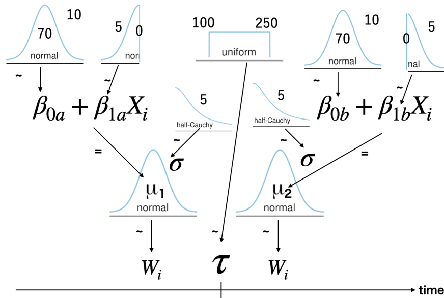
図 8.8 折線回帰モデル設計図
