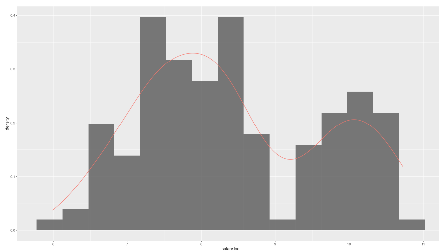
図 6.1 Tigers の選手年俸 (対数) の分布
