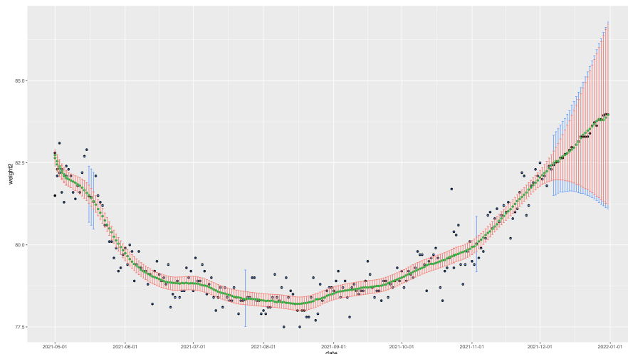
図 9.8 2階差分トレンドの予測
