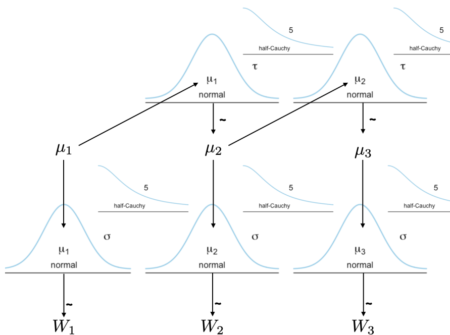
図 9.2 状態空間モデルの設計図
