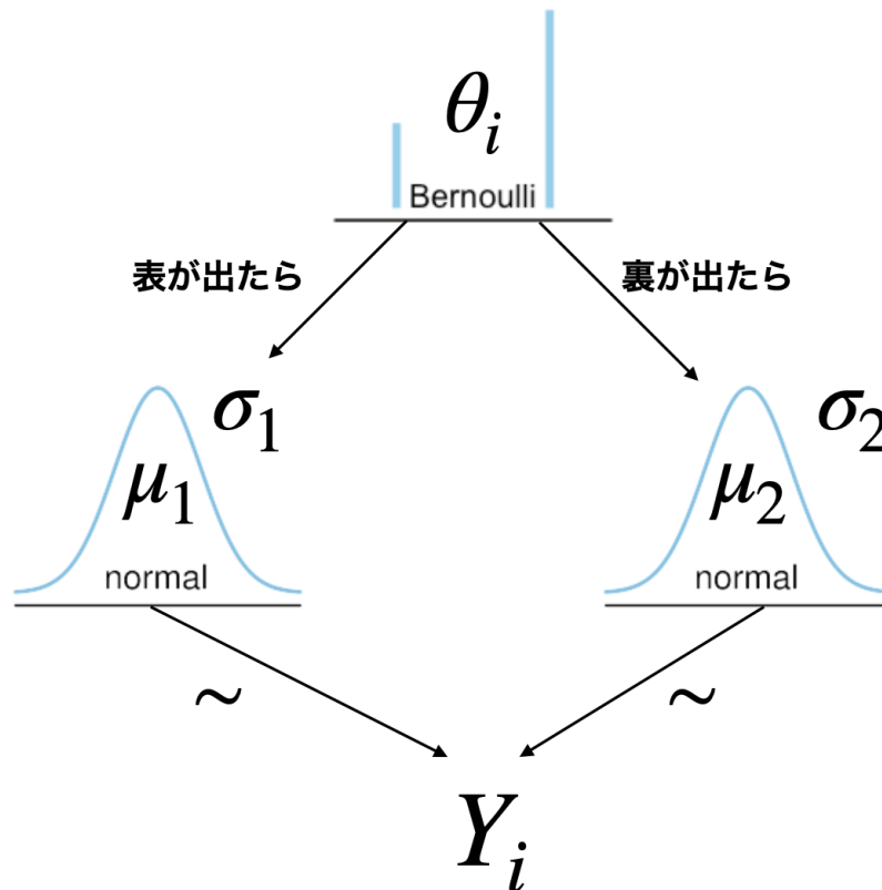
図 6.3 二つの正規分布からデータが出てくるモデル
