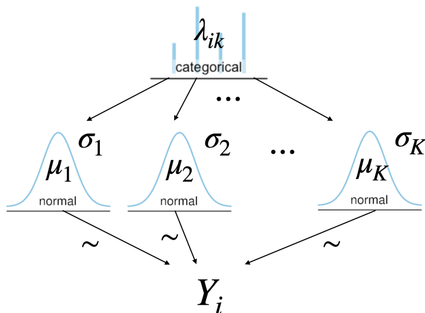
図 6.4 K 個の正規分布からデータが出てくるモデル
