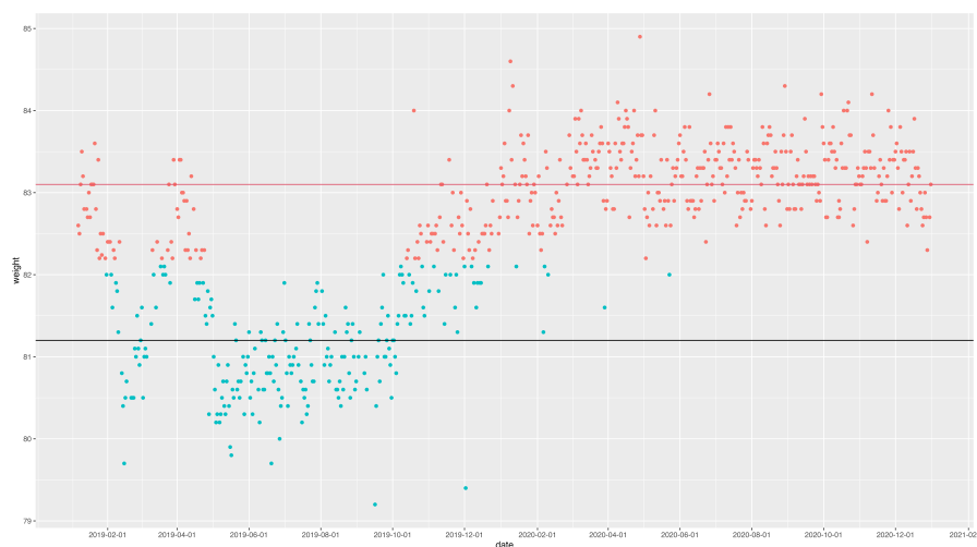
図 8.3 2つの体重のモード
