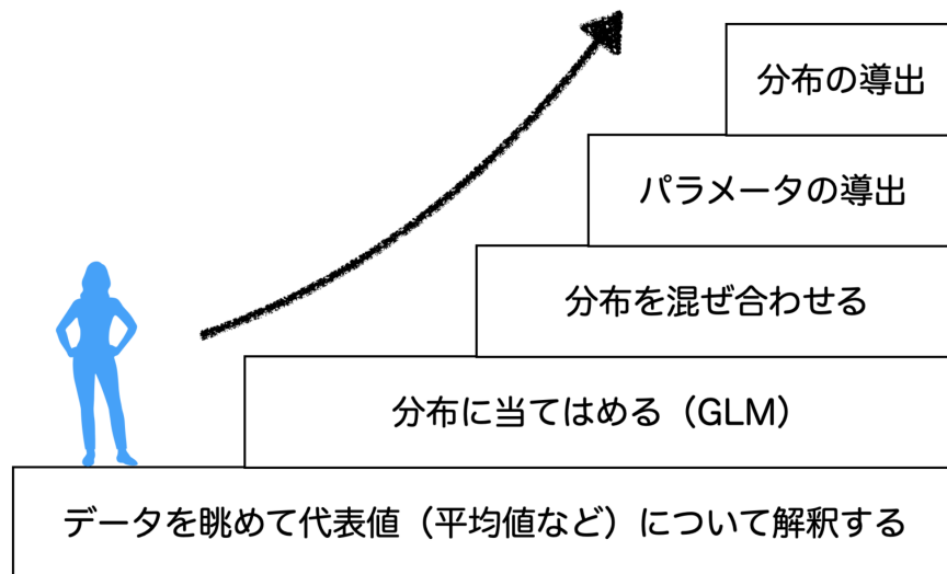
図 6.10 統計モデラーの道。浜田宏先生（東北大学）のアイデアをもとにイラスト化したもの
