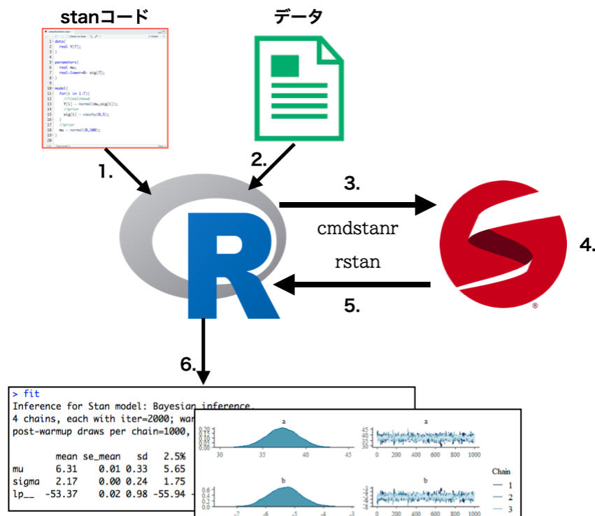
図 2.2 R/RStudio と Stan ファイルのやり取り
