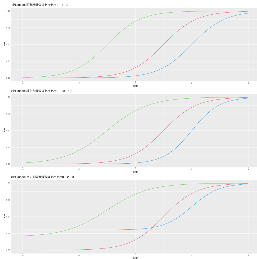
図 7.1 上から順に, 1, 2, 3 パラメータロジスティックモデル。どこがどう変わっていくか確認しておこう。
