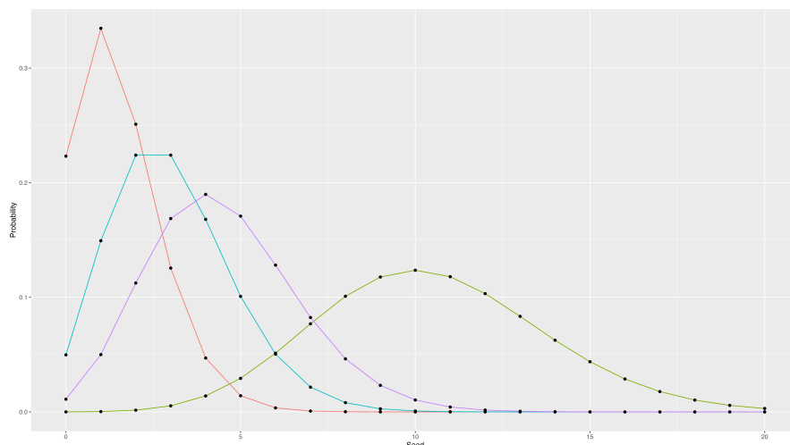
図 6.7 さまざまなポアソン分布。 \lambda は 1.5, 3, 4.5, 10.5 で描画
