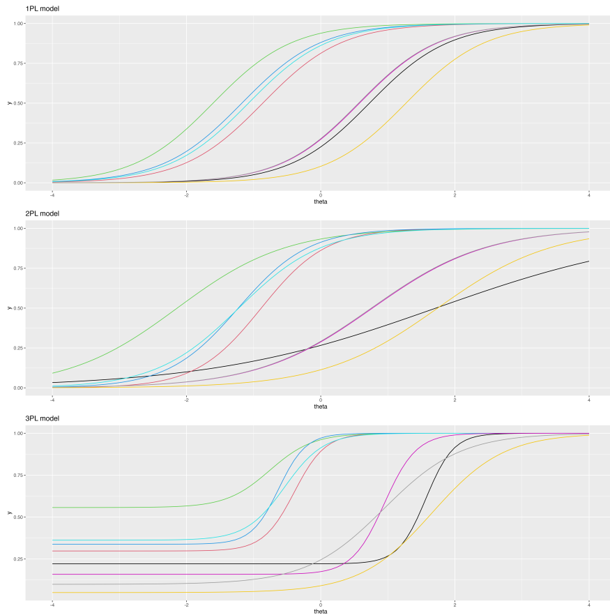
図 7.3 推定値を使って描いた各モデルの ICC
