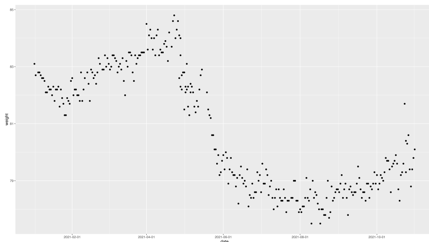
図 8.4 大きく変化したデータ
