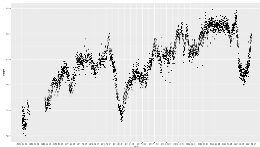
図 8.1 体重の時系列的推移
