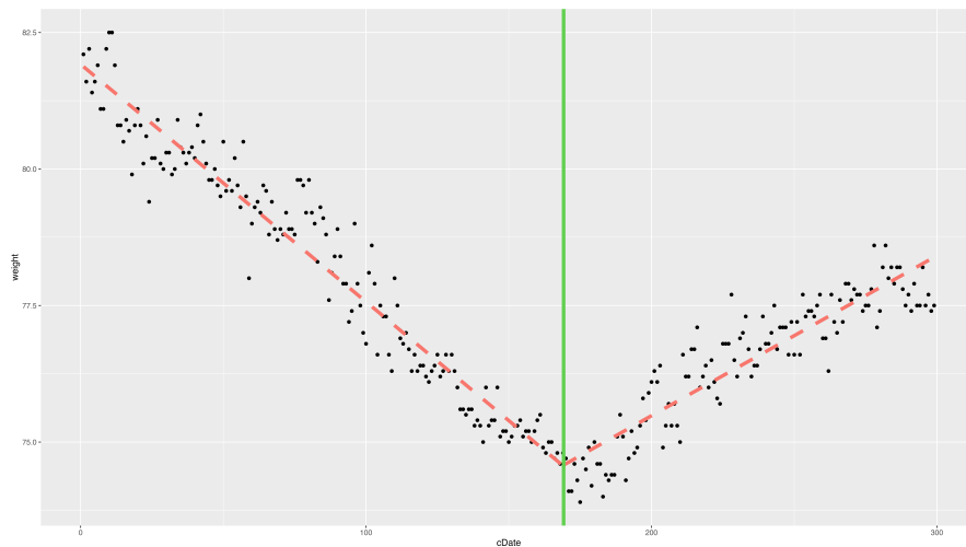
図 8.10 変化点を合わせた折線回帰モデル
