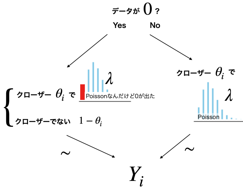
図 6.8 ポアソン分布との混ぜ合わせ
