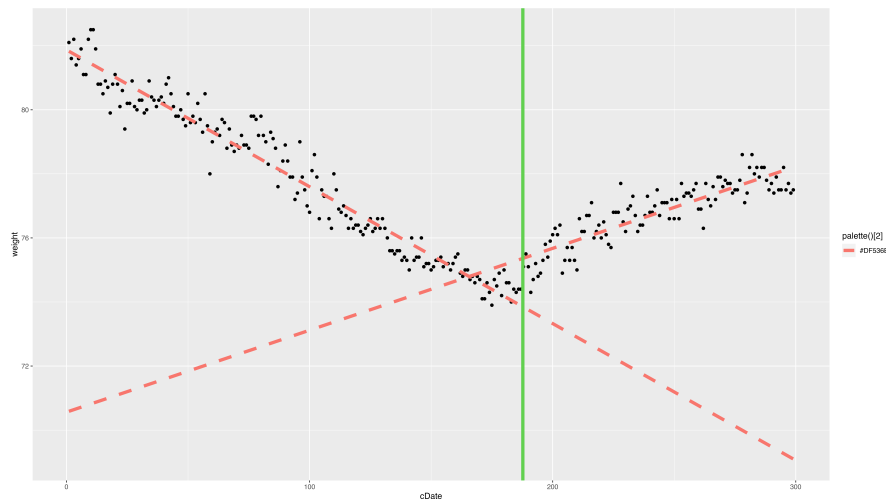
図 8.9 折線回帰モデル推定結果
