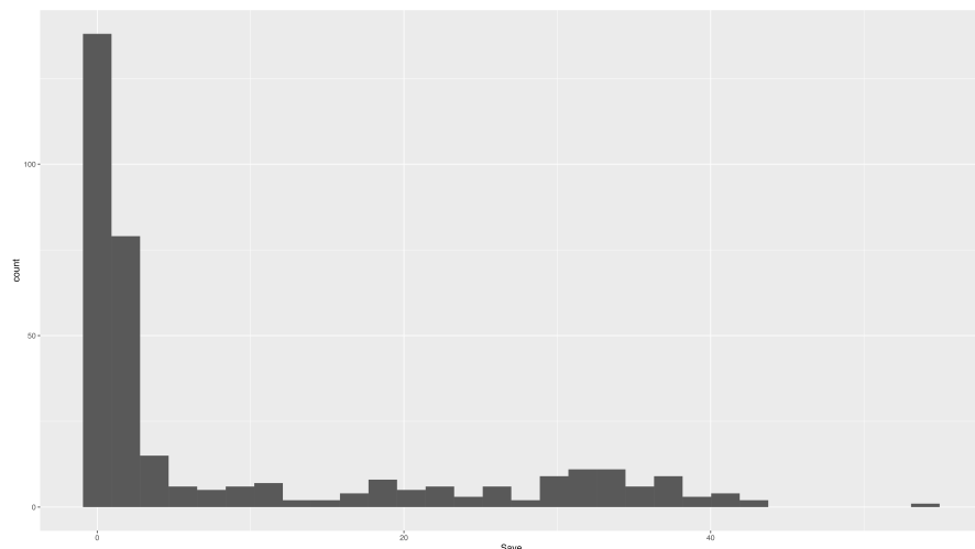
図 6.6 投手のセーブ数
