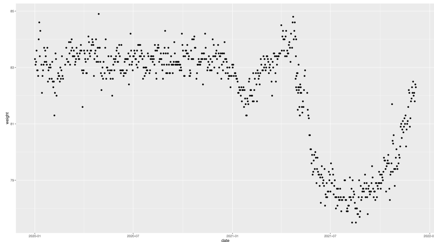
図 9.3 2020 年の体重変化
