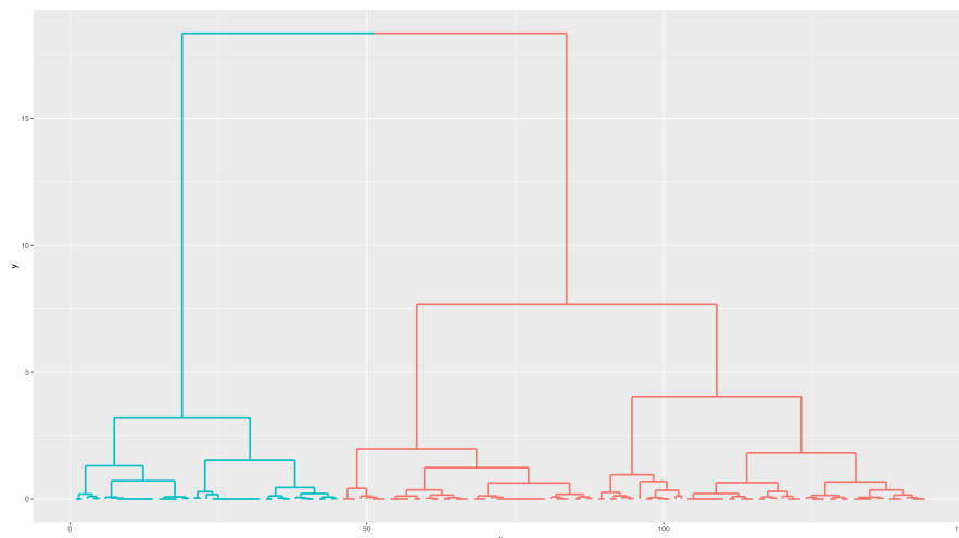
図 6.2 Tigers の選手を年俵で階層的クラスタリング (ウォード法による)
