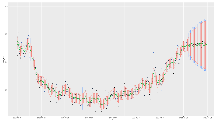
図 9.7 未来もある意味欠測値
