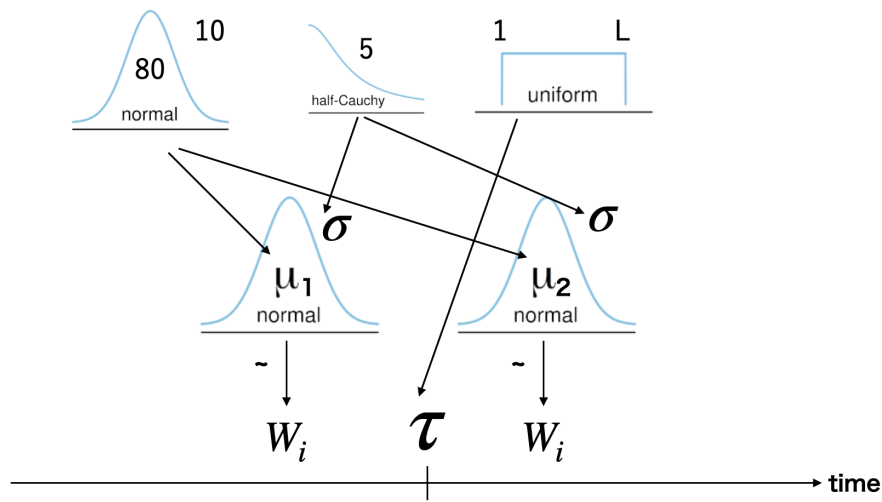
図 8.5 変化点検出のモデル設計図
