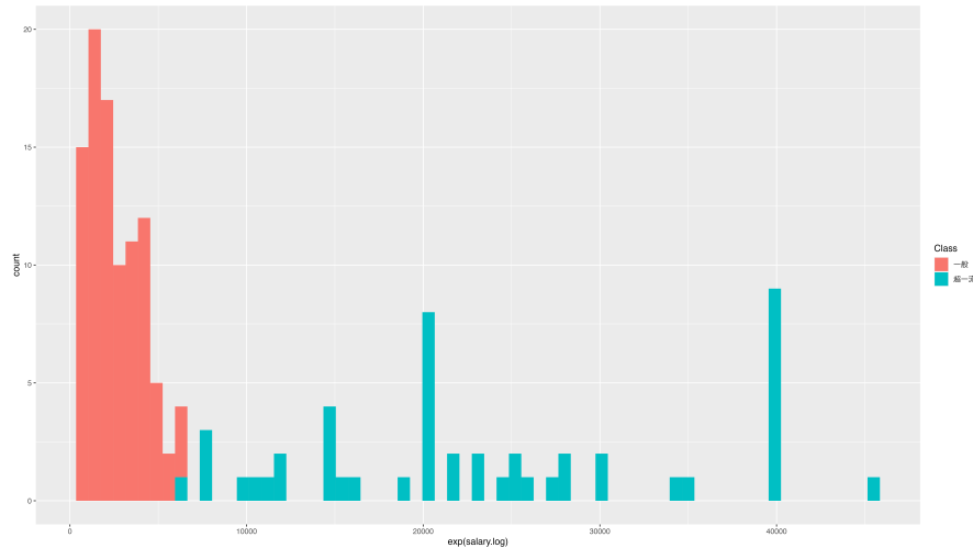
図 6.5 選手のクラスタリング
