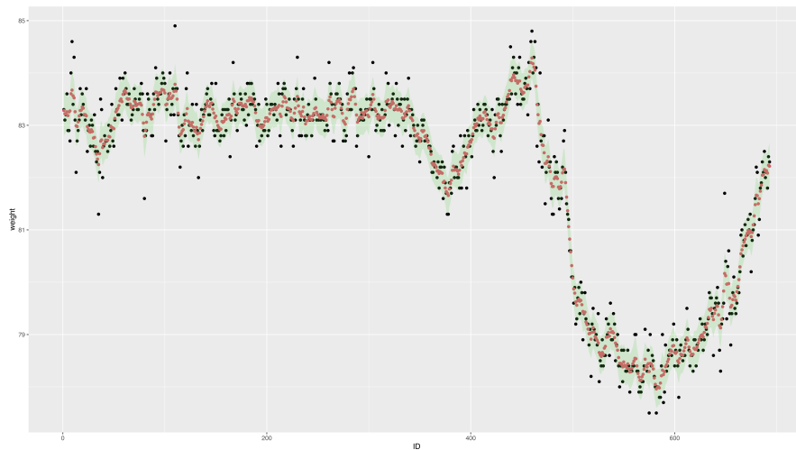
図 9.4 2020 年の体重変化をモデルで追跡してみた結果
