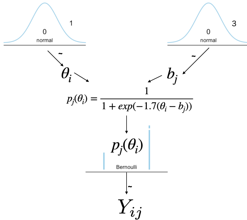
図 7.2 確率モデルとしての設計図。ロジスティック関数とベルヌーイ分布の組み合わせでテスト理論のモデルが表現できる。
